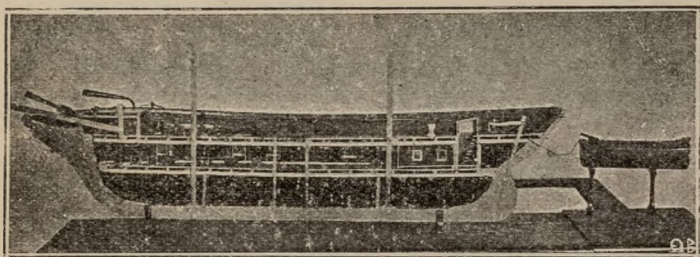
Τομὴ πυρπολικοῦ.
