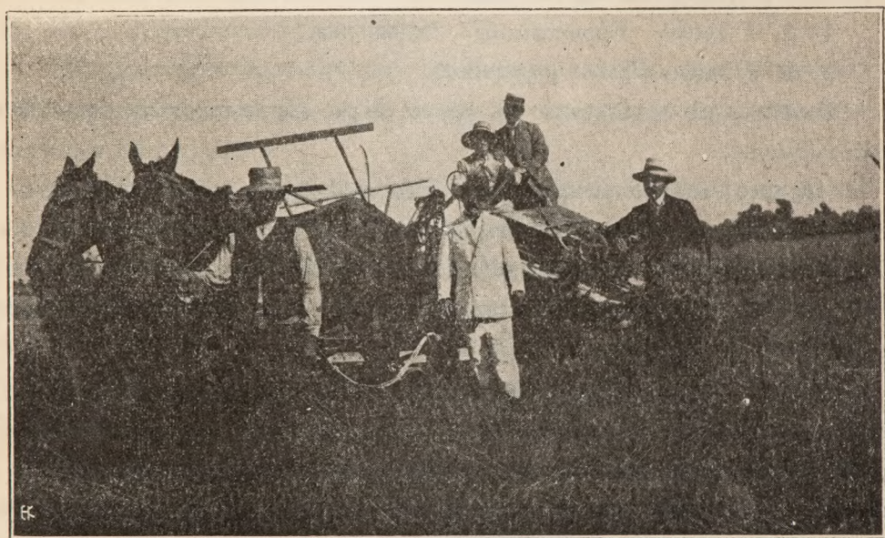
Ἡ αὐτοδευτικὴ μηχανὴ «Osborne» τὸ πρῶτον λειτουργήσασα ἐν τῷ νομῷ Αἰτωλίας καὶ Ἀκαρνανίας εἰς τὸ κτῆμα Σπυρ. Παπουτισοπούλου παρὰ τοῦ ἀγροκηπίου Μεσολογγίου.
